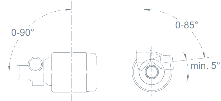
Målskitse Aquavent 6000SC ( U4856 )
