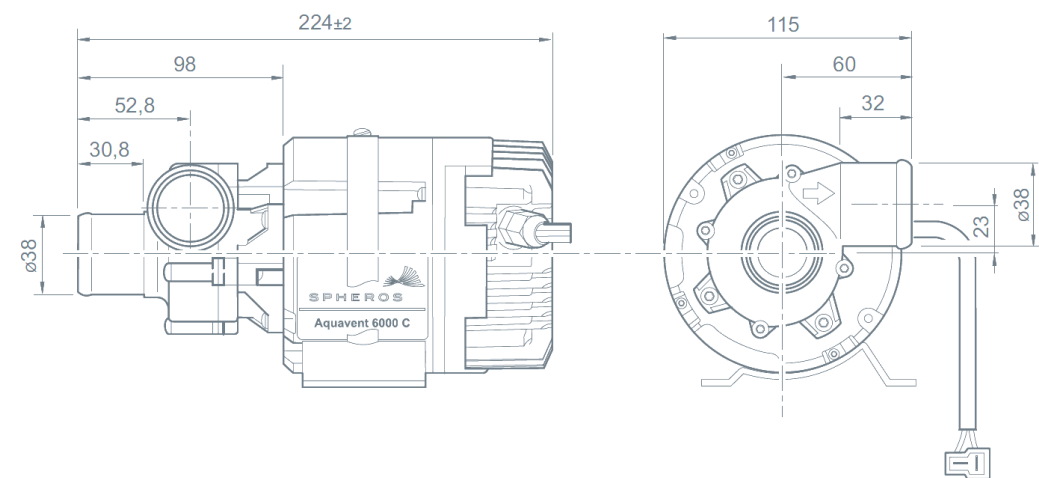
Målskitse Aquavent 6000C ( U4855 )
